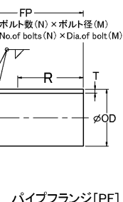
パイプフランジ[PF]
