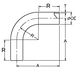
90° ロングエルボ[90LR]
