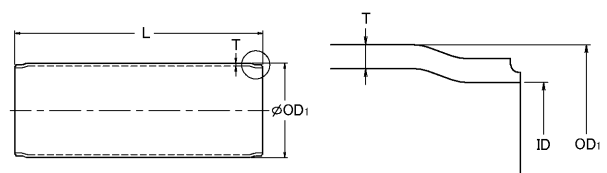
オーバーチューブ(タイプII) [D-OT]
