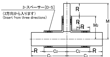
異径ティーズ[D-RT]
