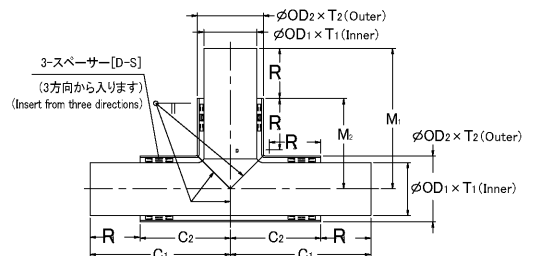
同径ティーズ [D-ET]
