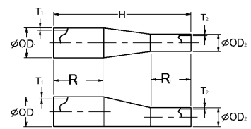
同心/偏心レジュューサー[RC][RE]
