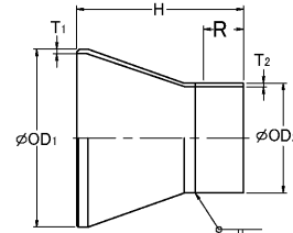
同心／偏心レジュースー [RC][RE]
